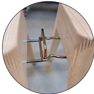
Bügel- Reihenverbindung
